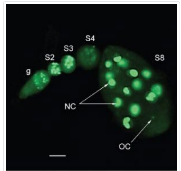
ADN fragmenté de cellules ovariennes de drosophile exposée aux ondes GSM 900 MHz. © Dimitris Panagopoulos
